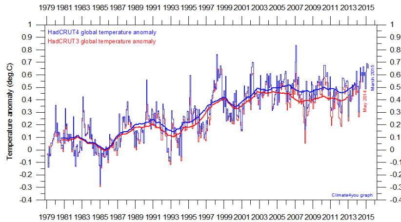
HadCRUT (land surface + ocean)
