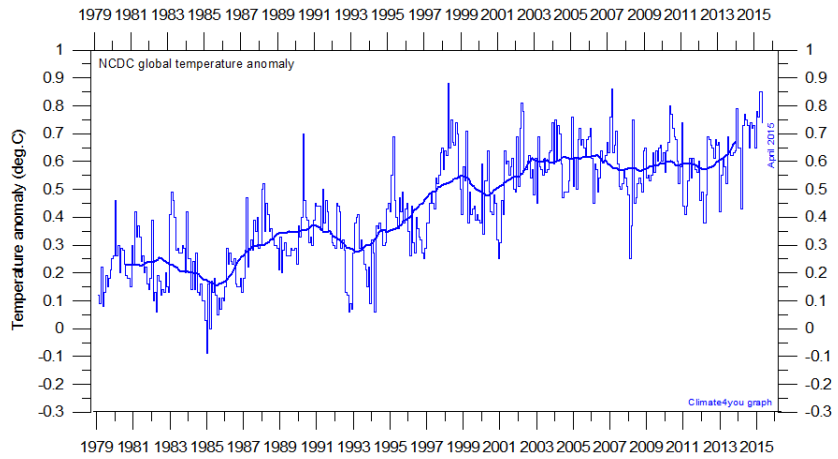
NDCG (land surface + ocean)
